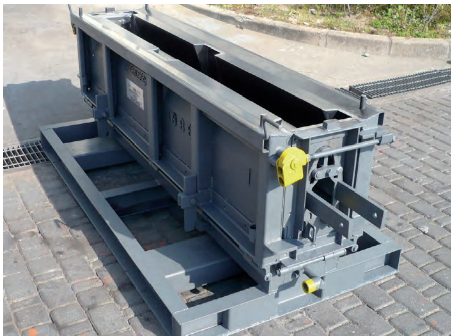
Рис. 5: Форма для производства яйцевидных дренажных лотков
