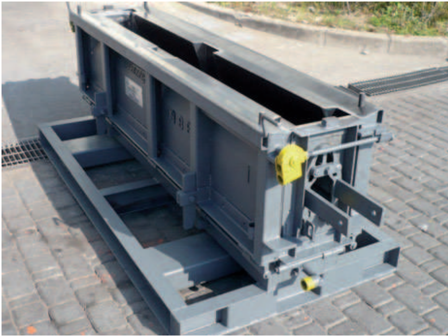
Abb. 5: Schalung für eiförmige Straßendrainagen
